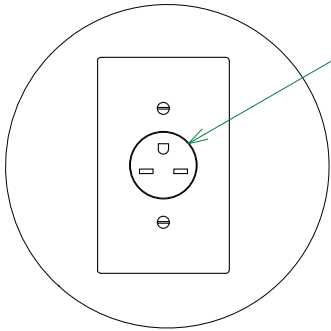
DETAIL 1-A RECEPTACLE DETAIL
